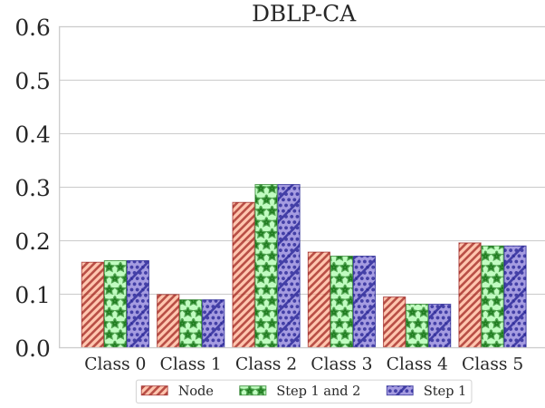
(d) Class distribution for DBLP-CA.
